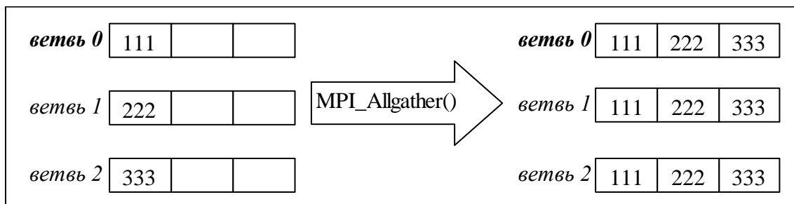
Рис. 29 Работа MPI_Allgather()
