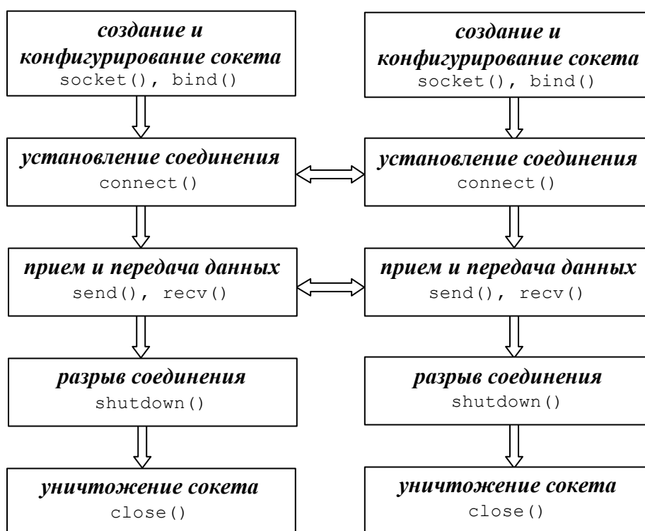
Рис. 21. Схема работы с сокетами с установлением виртуального канала
