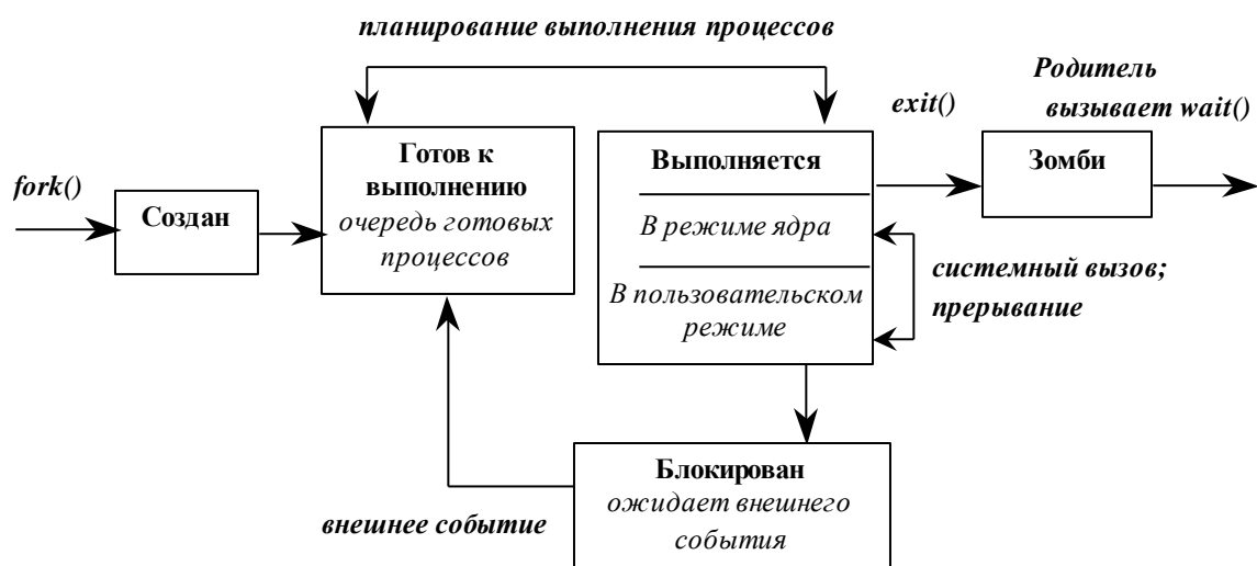
Рис. 12 Жизненный цикл процесса в ОС UNIX.
