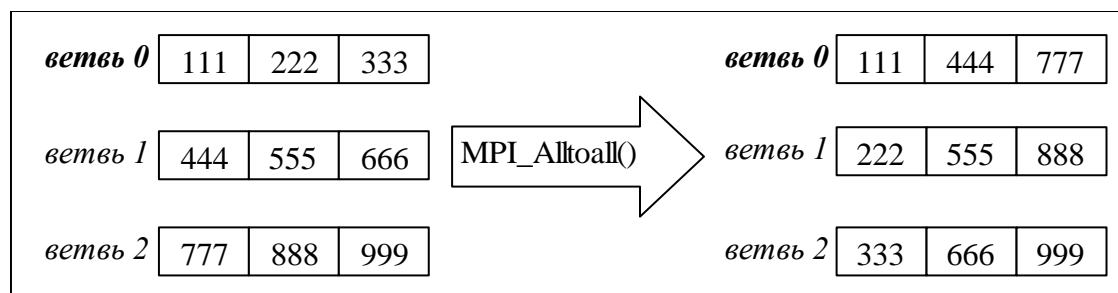
Рис. 30 Работа функции MPI_Alltoall()
