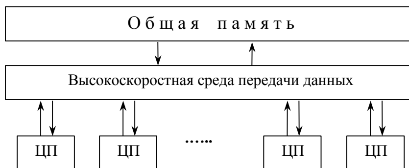
Рис. 27 Архитектура SMP.
