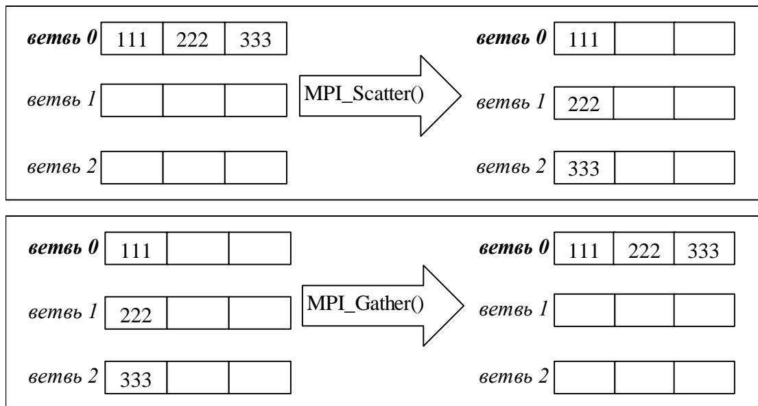
Рис. 28 Работа MPI_Scatter() и MPI_Gather()
