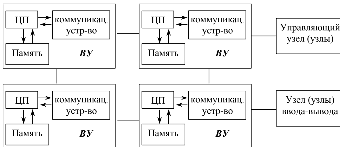
Рис. 26 Архитектура MPP.
